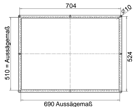
Einbaumaße Arbeitsplatte AK 6
