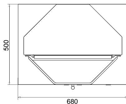
Grundmaße Thekengerät AK 5
