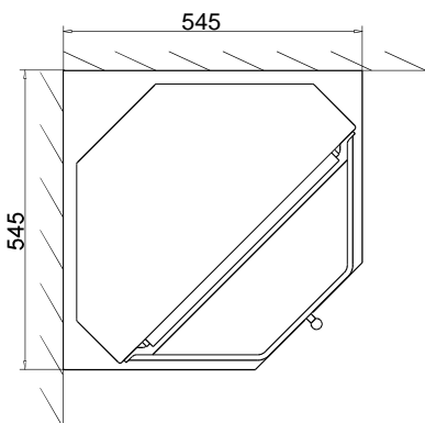
Grundmaße Eckgerät AK 4
